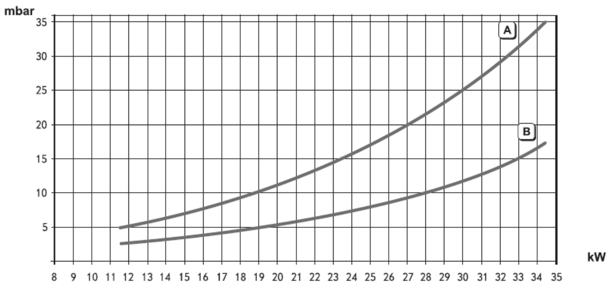
Рис. 13. График зависимости мощности котла от входного давления газа. A – сжиженный газ, B – природный газ.
