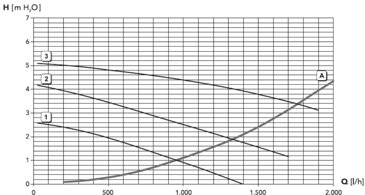
Рис. 12. Потери напора циркуляционных насосов. A – потери напора в котле; 1, 2 и 3 – скорость циркуляционного насоса
