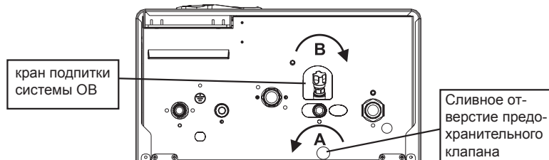
Рис. 6. – Кран для заполнения водой системы отопления (СО)
